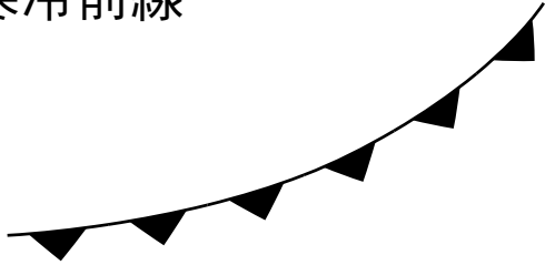
かんれいぜんせん 寒冷前線
