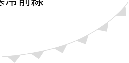
かんれいぜんせん 寒冷前線
