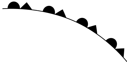
へいそくぜんせん 閉塞前線
