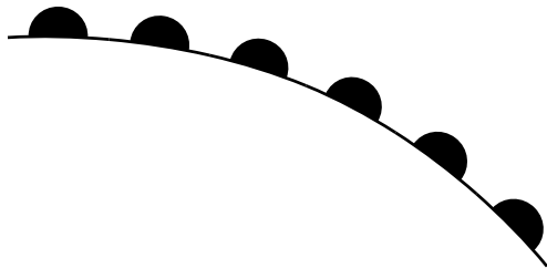
おんだんぜんせん 温暖前線
